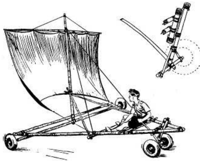
Land Yacht.
